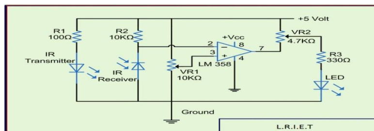
IR Sensor Circuit
